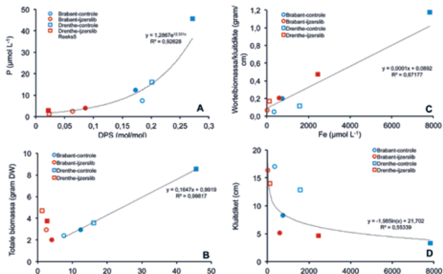
Figuur 4 (A) correlaties tussen de DPS (mate van P-verzadiging) en de concentratie P in het poriewater, (B) de concentratie P in het bodemvocht en de totale biomassa van H. lanatus , (C) de concentratie Fe in het bodemvocht en de ratio tussen de wortelbiomassa en de kluitdikte, en (D) Fe-concentratie in het bodemvocht en kluitdikte. Gesloten symbolen geven de waarden bij de hoge waterstand, open symbolen bij de lage waterstand. Gemiddelde waarden (n=3) zijn gegeven. De P-concentratie betreft de concentratie op het einde van de incubatieproef.
